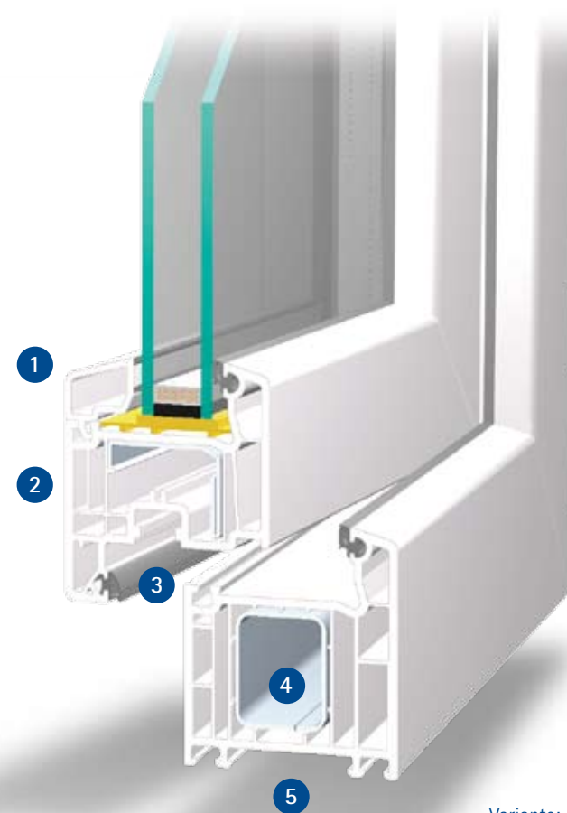
Variante: flächenversetzt
